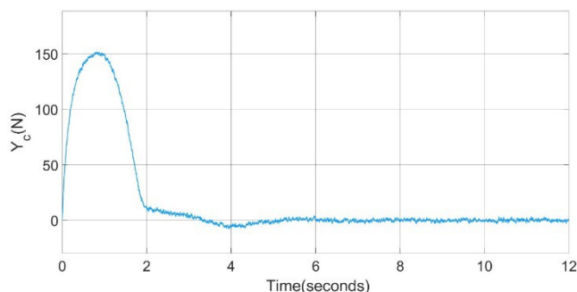
Figura 6 Resultados del ROV con L1 adaptativo; señal de control Y_c(N) calculada por el controlador
